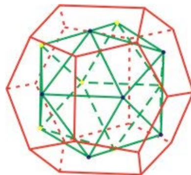
Dodekaeder
